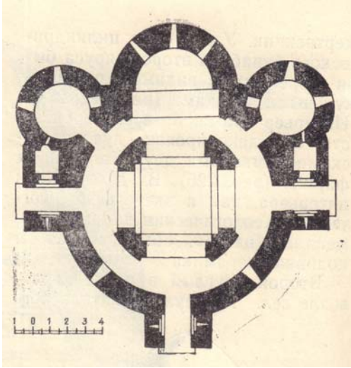
ՊՃ. 1 - Մամրուխի եկեղեցու հատակագիծը (ըստ Ախունդովի)
