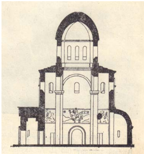
ՊՃ. 2 - Մամրուխի եկեղեցու կտրվածքը (ըստ Ախունդովի)
