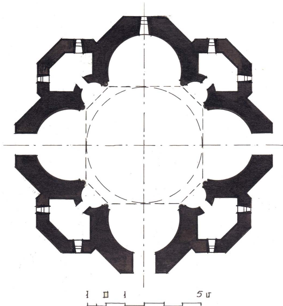
ՊՃ. 1 – Չախմուս եկեղեցու հատակագիծը (վերակազմություն՝ Տ. Մարությանի):
