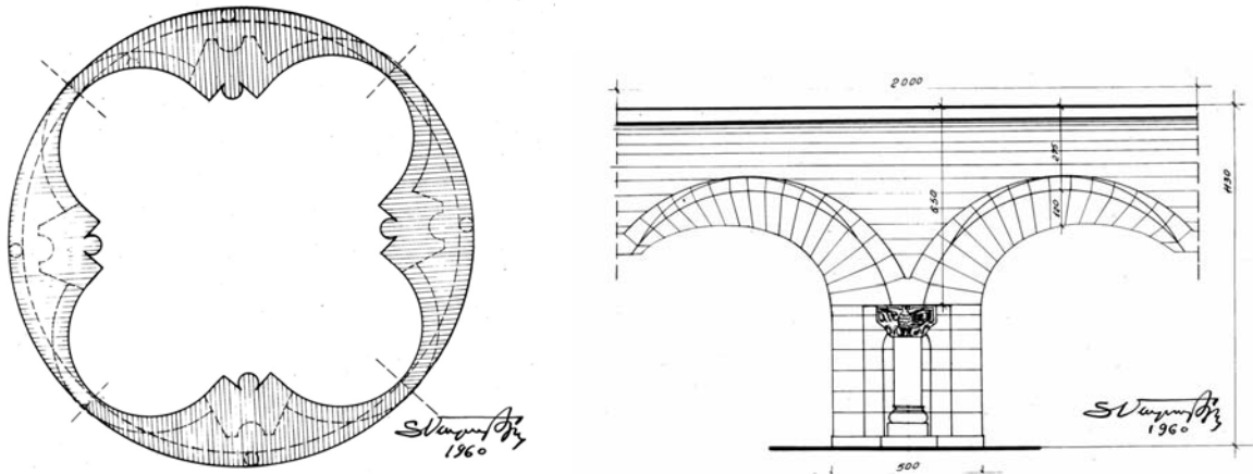
ՊՃ. 4-5 – Քարակրաբետոնակալուր բոլորաձև զանգվածի հաստակազիծը (ձախից) և տեսքը (վերակազմություն՝ Ս. Մարտիրոսյանի)
