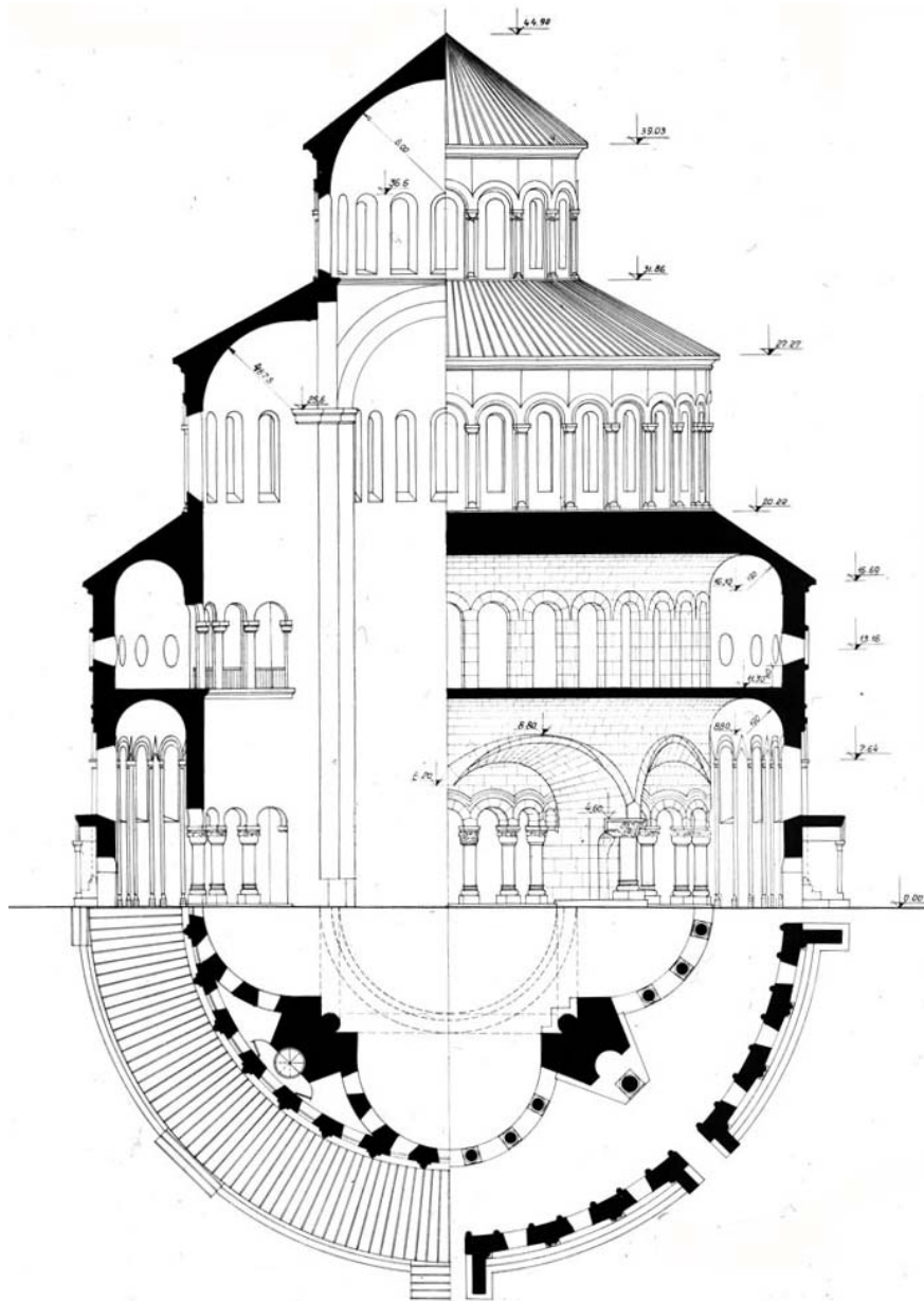
Գծ. 2 – Զվարթնոց. Պայմանական կտրվածք (վերակազմություն՝ Ս. Մարությանի)
