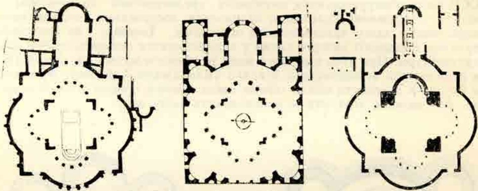
Рис. 2. Планы Селевкии, Босры, Апамен.
