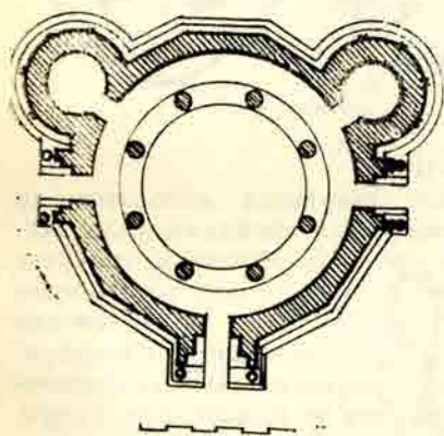
Рис. 1а. План Килисадага.
