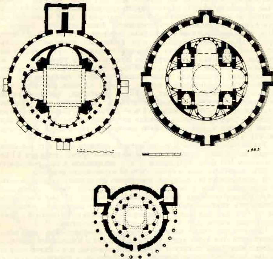
Рис. 3. Планы Звартноца, Банака, Лекита.
